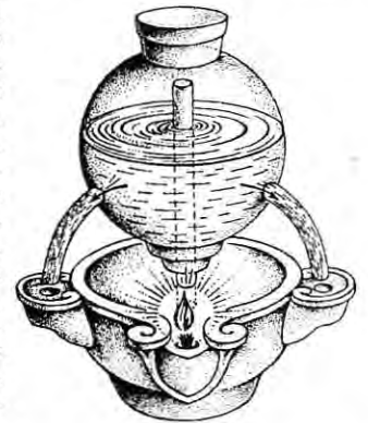
Светильник с автоматическим доливом жидкого топлива.
