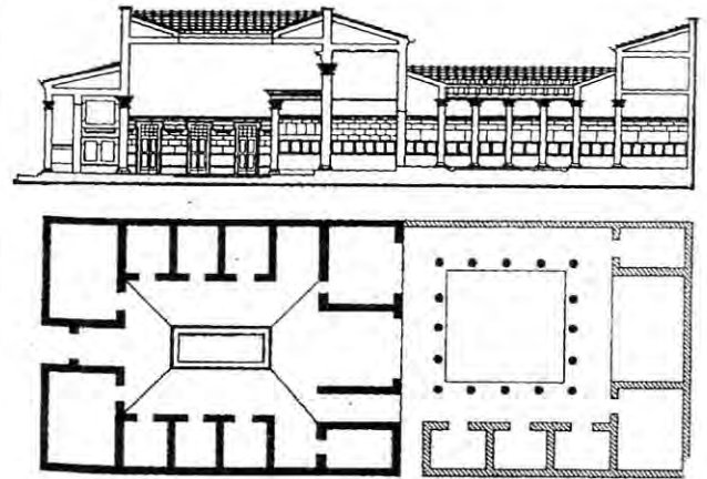
Планировка греческого дома.
