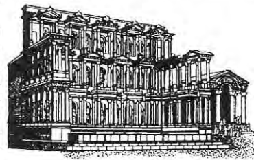
Милетский Нимфей.
