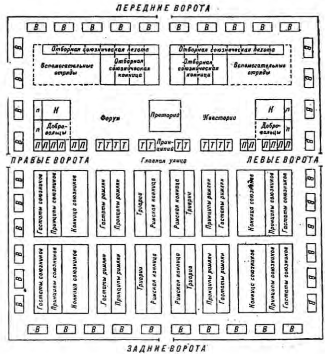
Римский лагерь.
