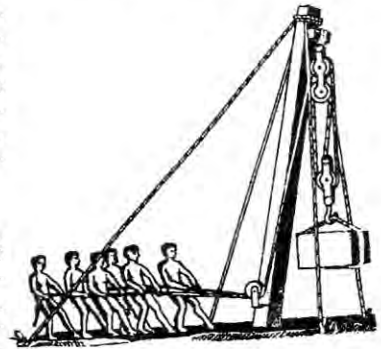
Кран.
