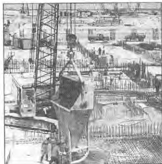
Строительство главного корпуса Ровенской атомной электростанции. 1977 г.
