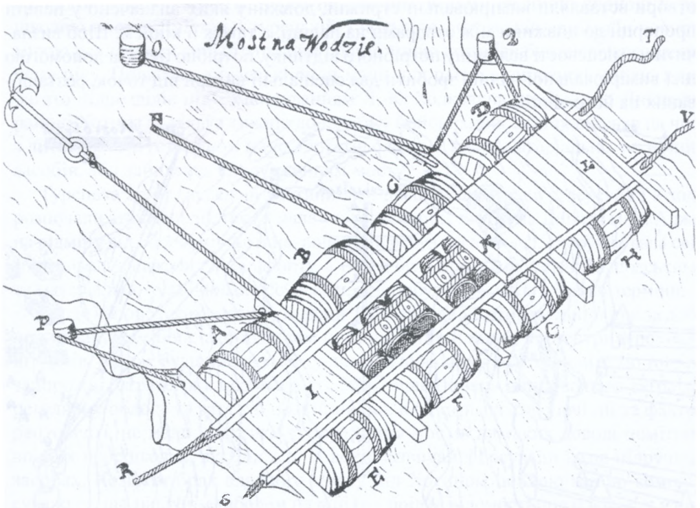
Схема спорудження наплавного мосту на бочках. Мал. А. делла Аква. 1635 р.
