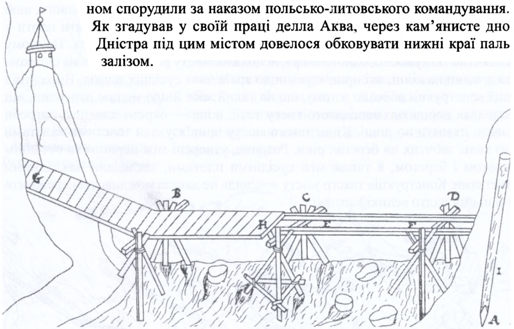
Схема спорудження мосту на кобилицях (козлах).
