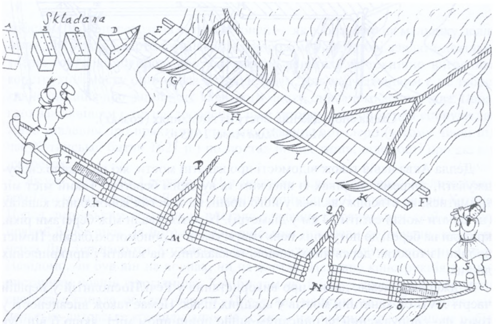
Схема спорудження наплавного мосту на човнах та плотах.
