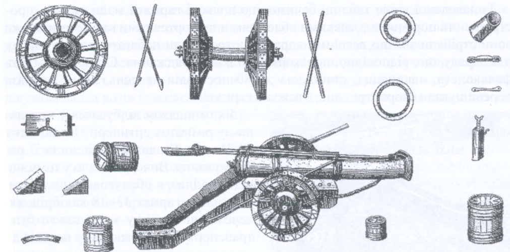
Картауна та принадлежності. Малюнок 1616 р.
