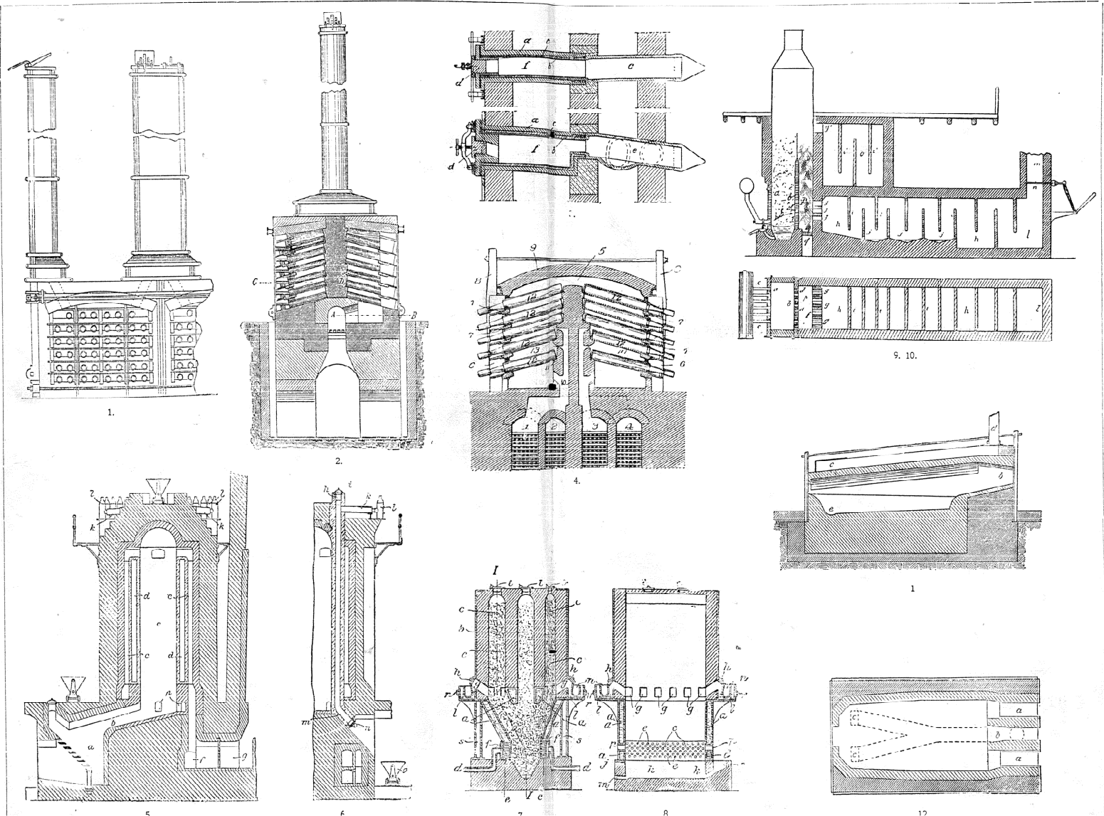
1, 2—Бельгийскія ретортныя печи. 3—Ретортная печь Бабэ и Трикара. 4—Ретортная печь Нейрентера. 5, 6—Муфельная печь Францисци. 7, 8—Шахтная печь Аристронга. 9, 10—Шахтная печь Себилло. 11, 12—Печь для рафинирования Ц. Брокгауз и Ефронъ, „Энцикл. Слов.“.
