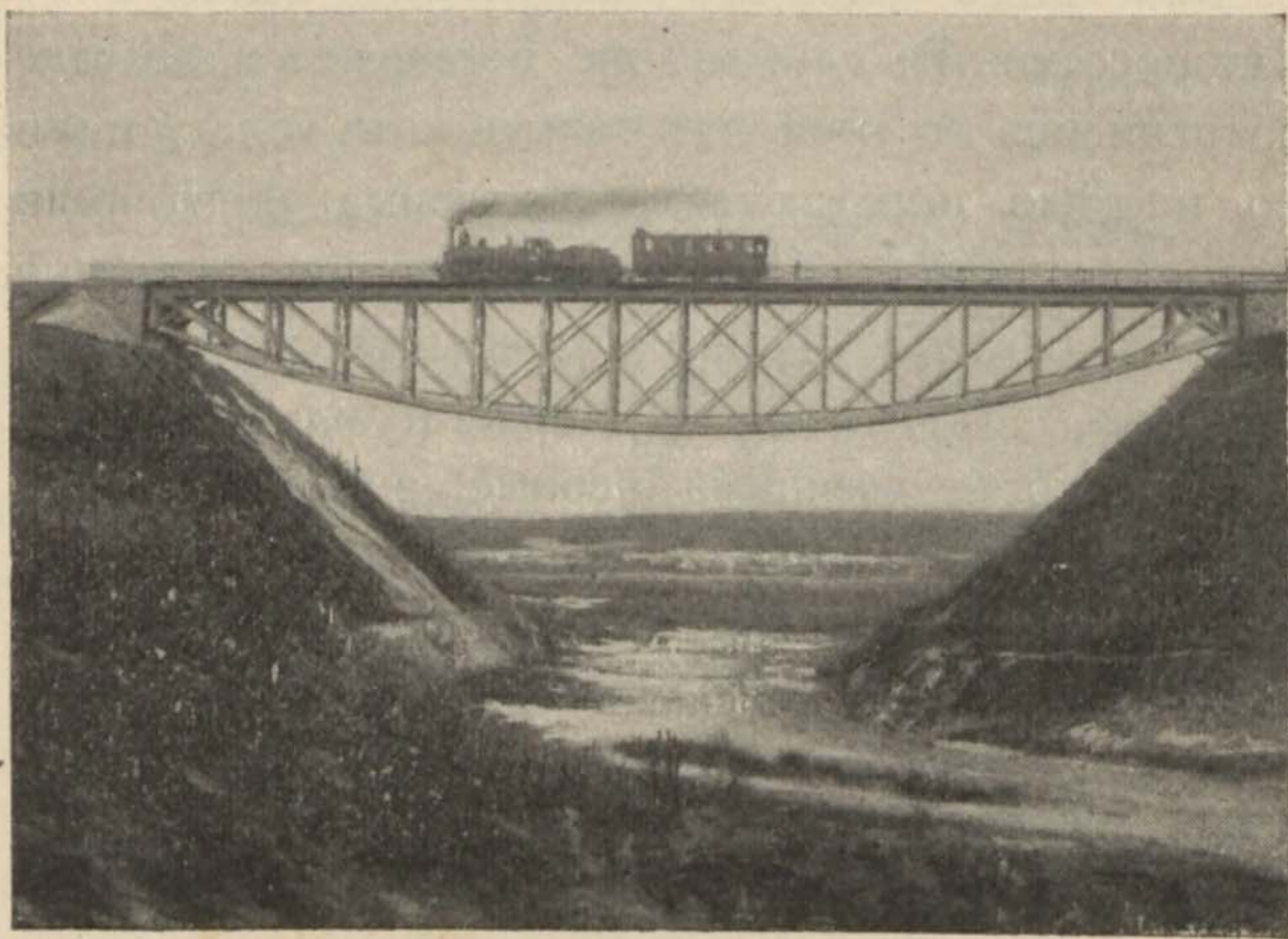
Мостъ на рѣкѣ Калфѣ.
