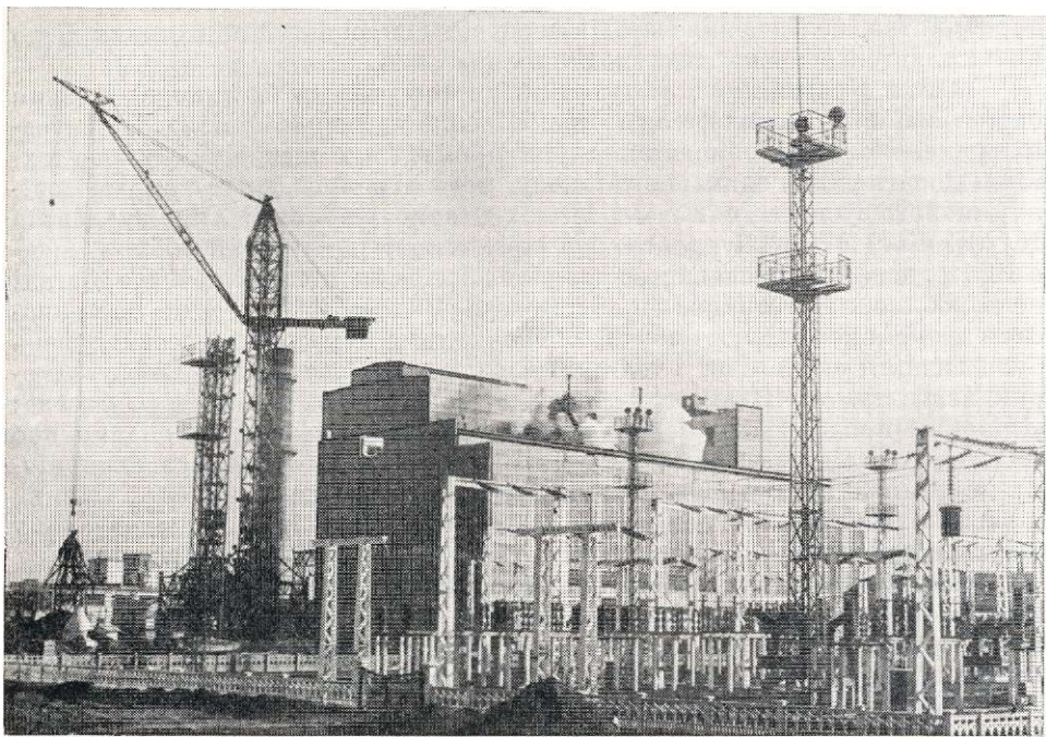
Загальний вигляд Сімферопольської ДРЕС ім. В. І. Леніна, вперше в СРСР повністю змонтованої із залізобетонних конструкцій і деталей (1958 р.).
