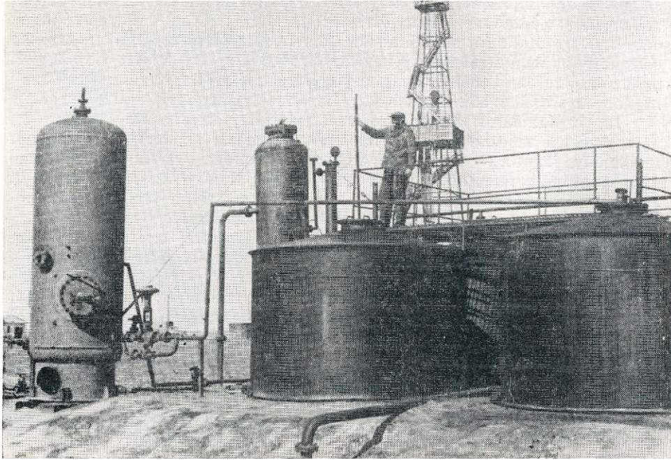
Групова установка для збирання нафти і газу на нафтопромислі (с. Радченки Миргородського району Полтавської області, 1955 р.).
