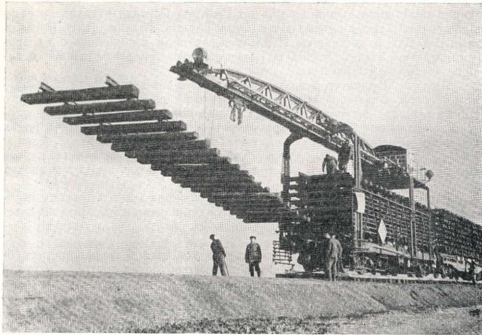
Новий тип шляхоукладача інженера Платонова на будівництві залізниці Федорівна—Каховка (1952 р.).
