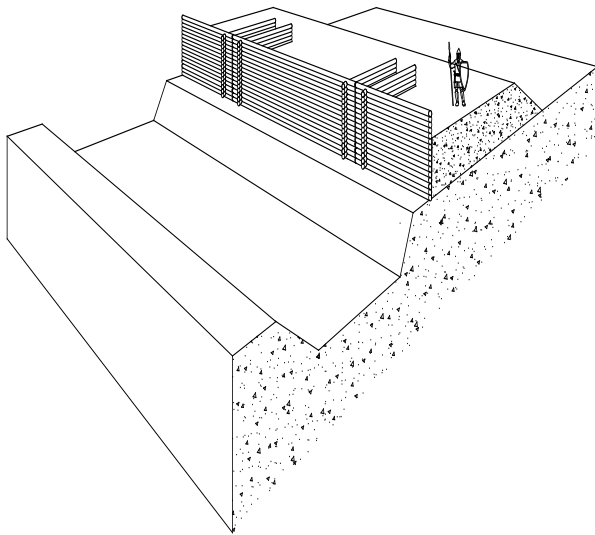
Ил. 7. Реконструкция оборонной стены городища из трёхстенного сруба на первом этапе строительства. Рисунок В. И. Лукьянченко.
