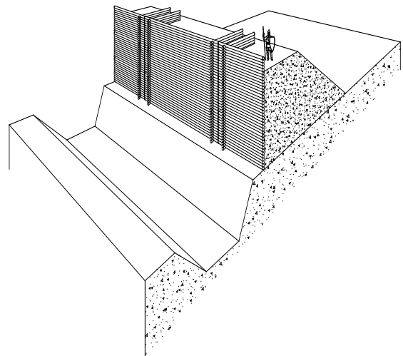
Ил. 8. Реконструкция оборонной дерево-земляной стены из трёхстенного сруба на втором этапе строительства. Рисунок В. И. Лукьянченко.
